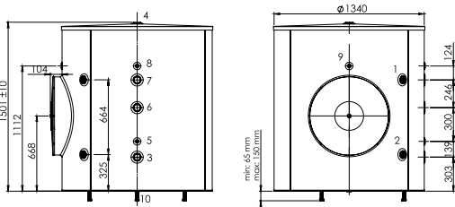
LCT INOX 1.500
