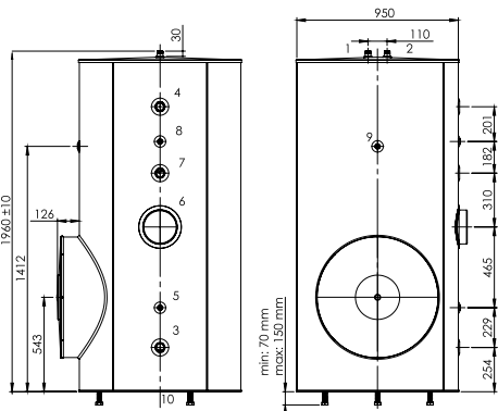
LCT INOX 1.000
