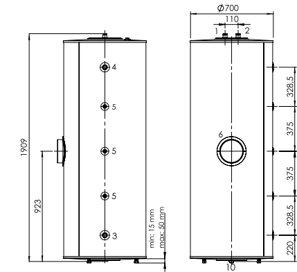
LCT INOX 500
